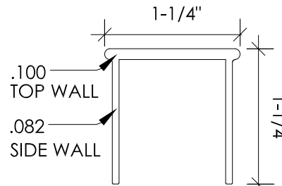
PICKET DETAIL SCALE: 3" = 1'-0"
